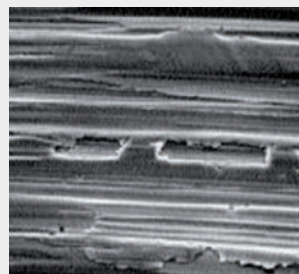
Ingrandita fino a 1500 volte, la superficie di un cuscinetto nuovo appare liscia.
